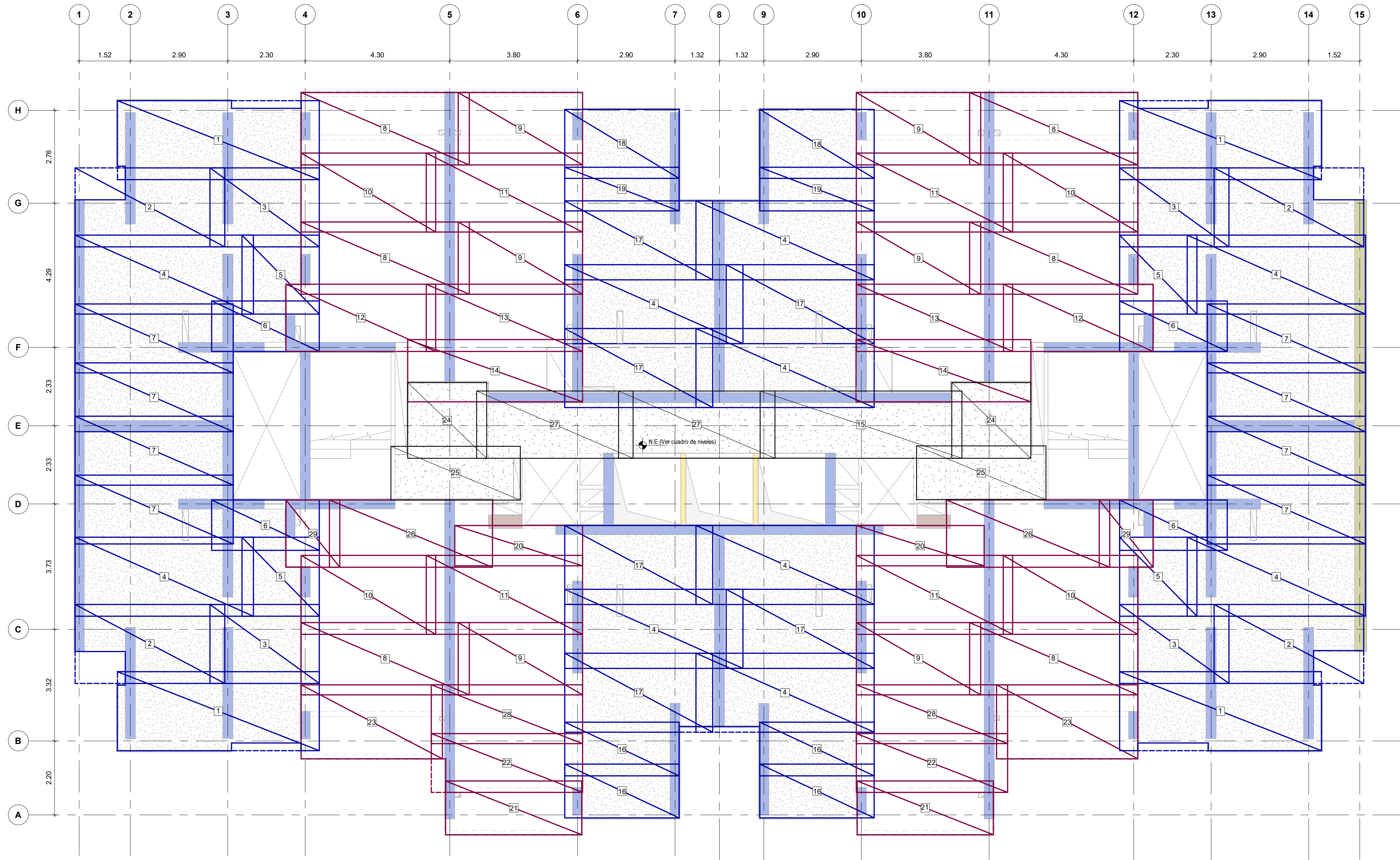
PLANTA DE REFUERZO INFERIOR PISO TIPO 1 ( PISO 3 A PISO 15) Escala 1 : 75
