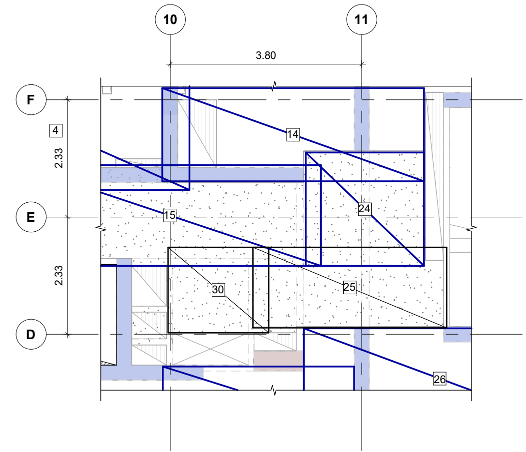
PLANTA DE REFUERZO INFERIOR PISO 14 Y PISO 15 Escala 1 : 75
